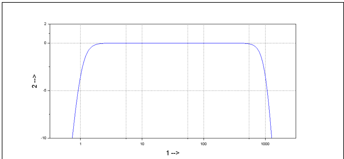
図2：典型的な周波数応答1 Hz～1000 Hz
