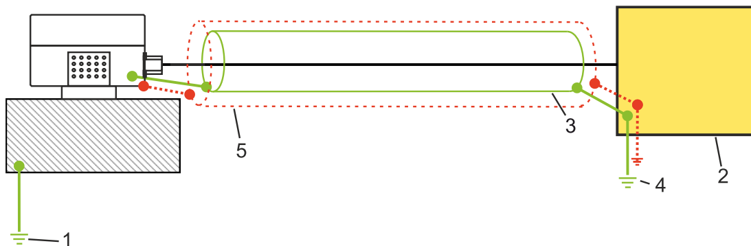
図13 : 接地コンセプトHE205
