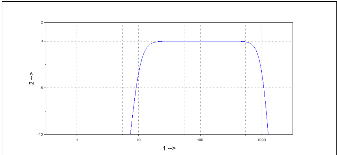
図1：典型的な周波数応答10 Hz～1000 Hz
