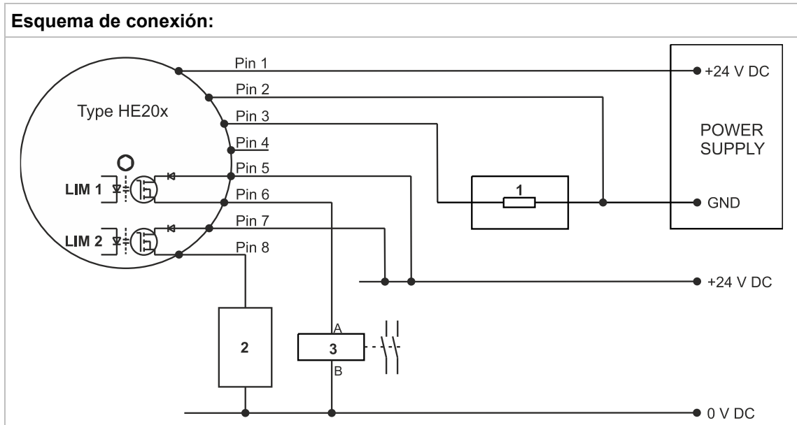
Fig. 6: Esquema de conexión
