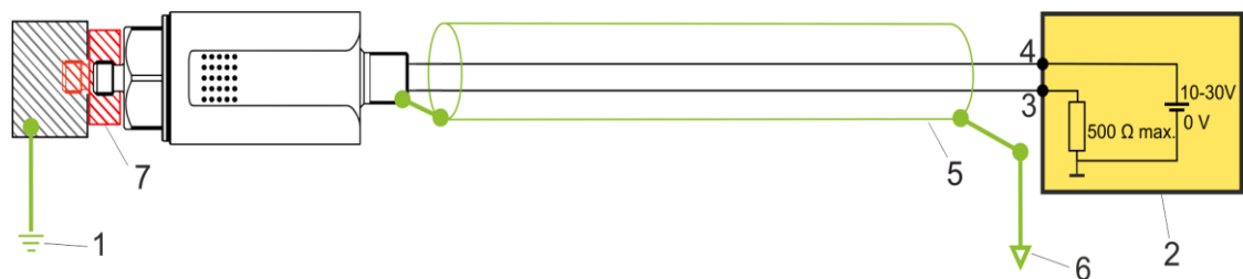
Fig. 11: Alternativt jordingskonsept
