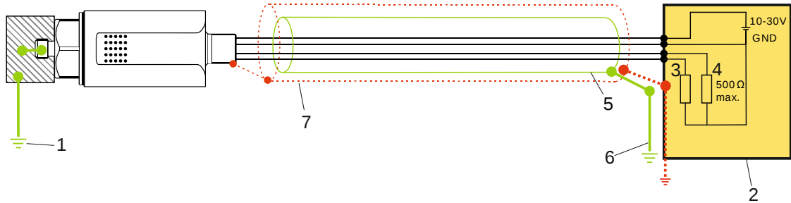
Şekil 10: Standart topraklama konsepti
