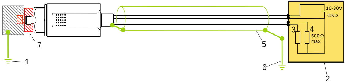
Şekil 11: Alternatif topraklama konsepti
