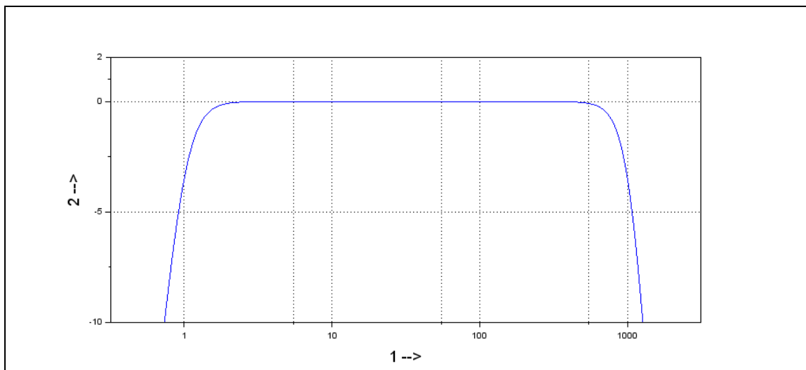
Fig. 7: Resposta de frequência típica de 1 Hz a 1000 Hz
