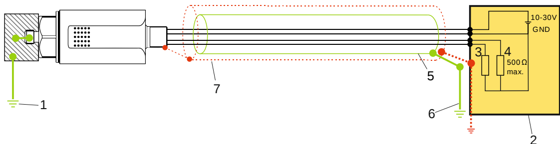
Afb. 10: Standaard-aardingsconcept
