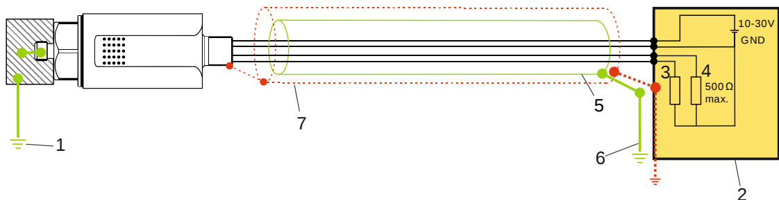
Fig. 10: Concepto estándar de puesta a tierra
