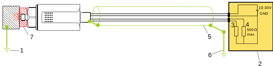
Fig. 11: Concepto de puesta a tierra alternativo
