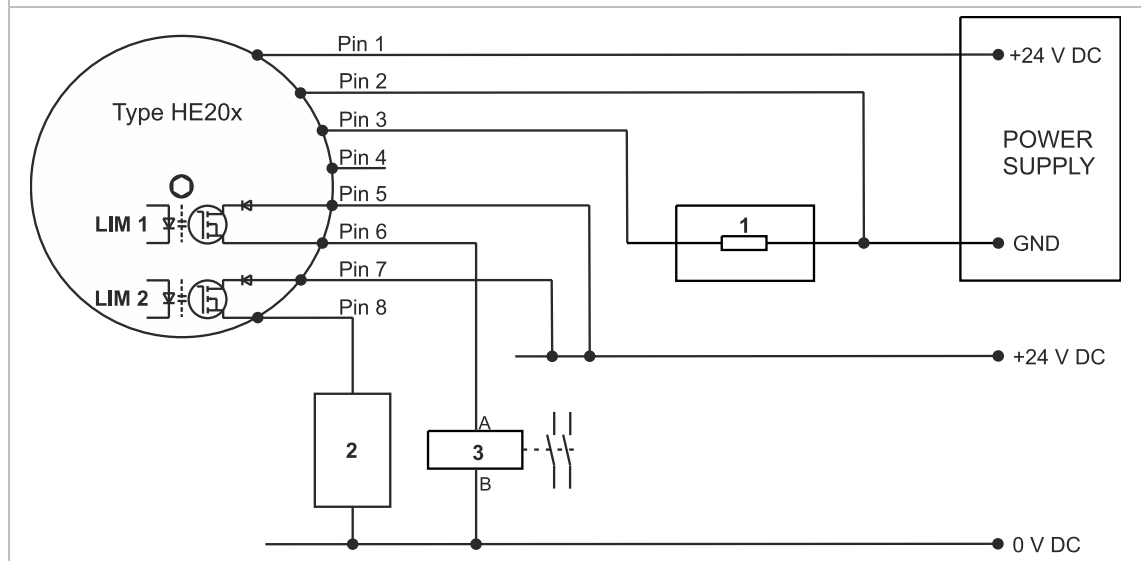
图 6：接线图
