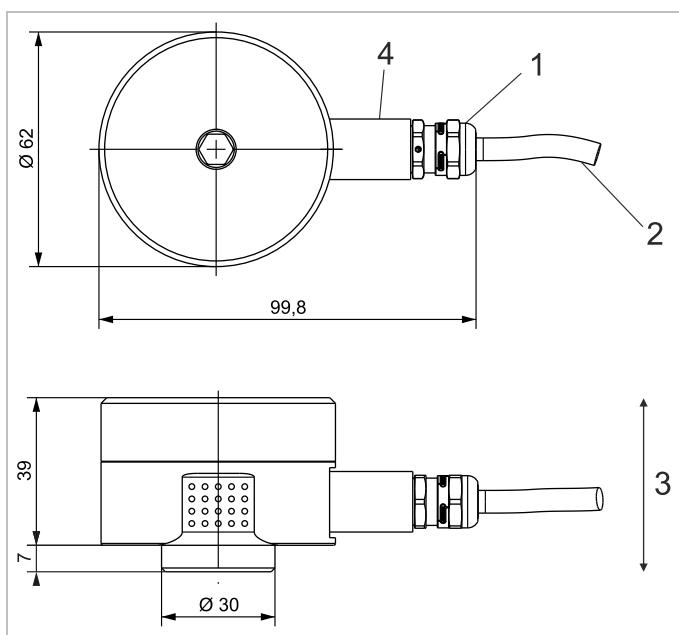
图 5：带集成式电缆和金属保护软管夹套底座的外壳
