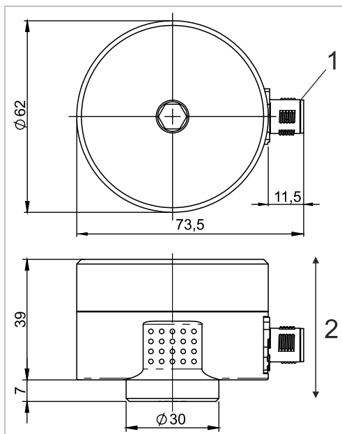
图 3：带 M12 插塞连接器的外壳
