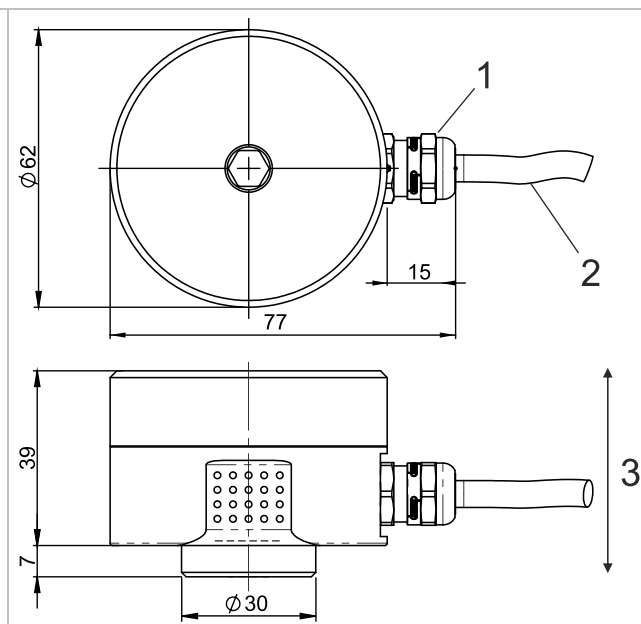
图 4：带集成式电缆的外壳
