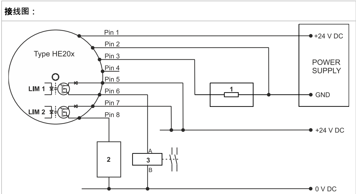
图 1：接线图
