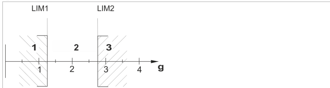
图 2：窗口功能
