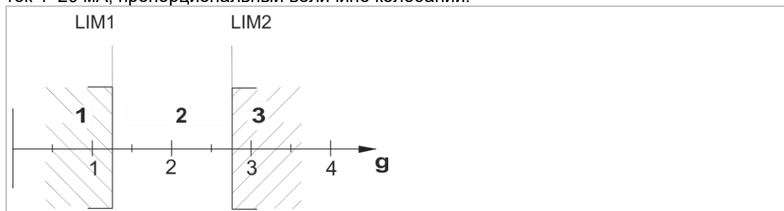
Рис. 2: Функция окна
