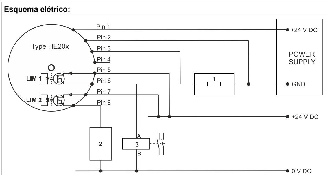
Fig. 1: Esquema elétrico
