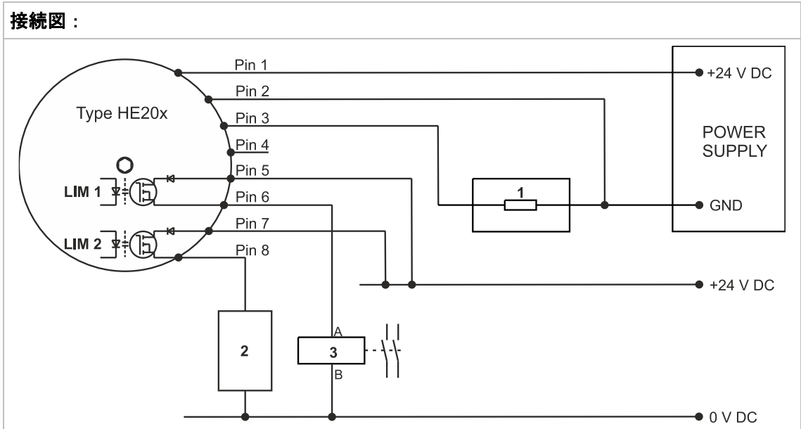
図1：接続図
