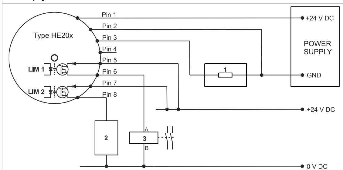
Obr. 1: Plán zapojení
