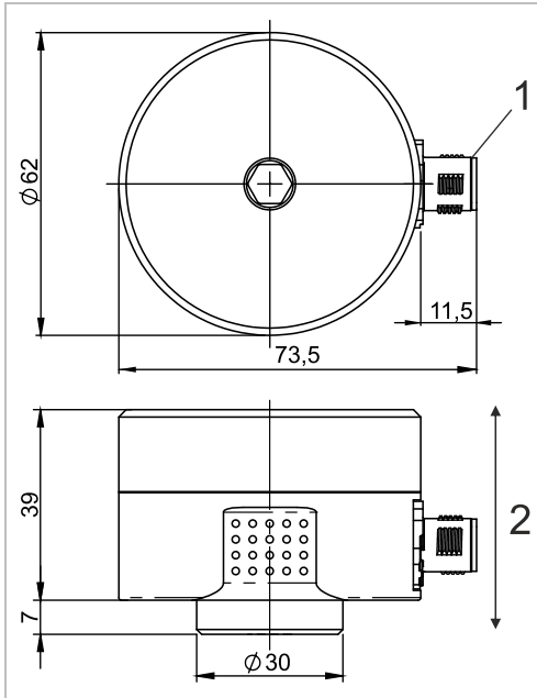
Şekil 4: Muhafaza, M12 soket bağlantısı ile
