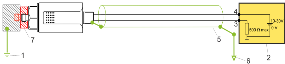
Afb. 11: Alternatief aardingsconcept
