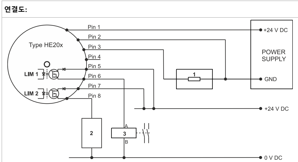
그림 6: 연결도
