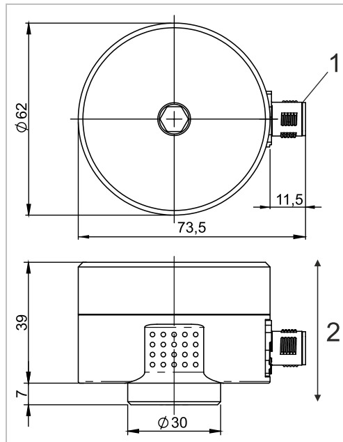
그림 3: M12 커넥터가 있는 하우징
