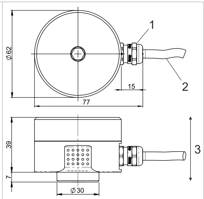
그림 4: 케이블이 내장된 하우징
